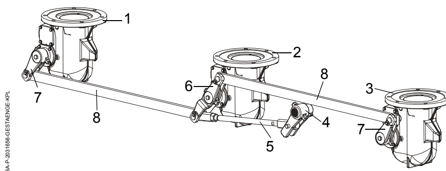
Varillaje del interruptor; vista de conjunto
