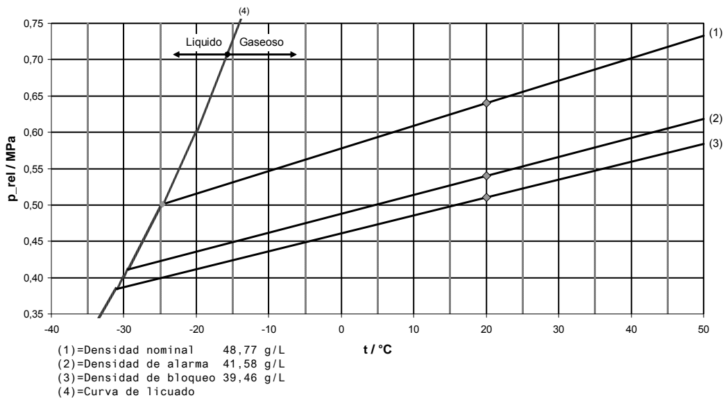
Curva de presión de SF 6 -30°C (ND =0,64 MPa [p e ] / UW1=0,54 MPa [p e ] / UW2=0,51 MPa [p e ])
